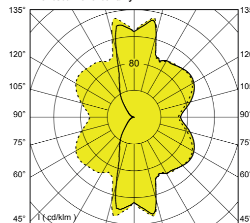
Lichtstärkeverteilung
