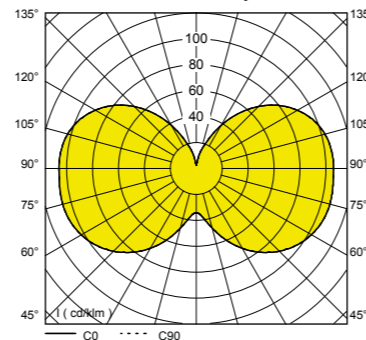
Lichtstärkeverteilung
