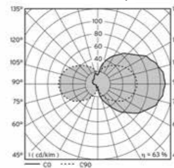
Lichtstärkeverteilung
