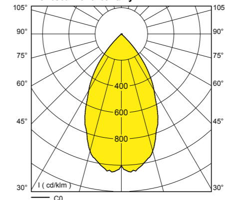
Lichtstärkeverteilung
