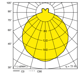
Lichtstärkeverteilung
