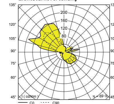
Lichtstärkeverteilung
