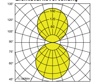
Lichtstärkeverteilung
